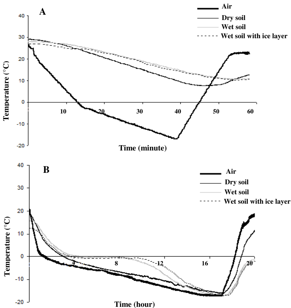
شکل ۲- مقایسه دمای خاک خشک، خاک مرطوب و همان خاک مرطوب با پوشش یخ در زمان کاهش دمای محیط تحت برنامه اول: سرعت کاهش دما 1\text{ }^{\circ}\text{C}/\text{min} تا دمای -15\text{ }^{\circ}\text{C} و سپس بلافاصله افزایش تا دمای +25\text{ }^{\circ}\text{C} (A) و برنامه دوم: سرعت کاهش دما 0.01\text{ }^{\circ}\text{C}/\text{min} تا دمای -15\text{ }^{\circ}\text{C} درجه سلسیوس، ۲ ساعت در دمای -15\text{ }^{\circ}\text{C} سپس افزایش به دمای +25\text{ }^{\circ}\text{C} درجه سلسیوس (B).
