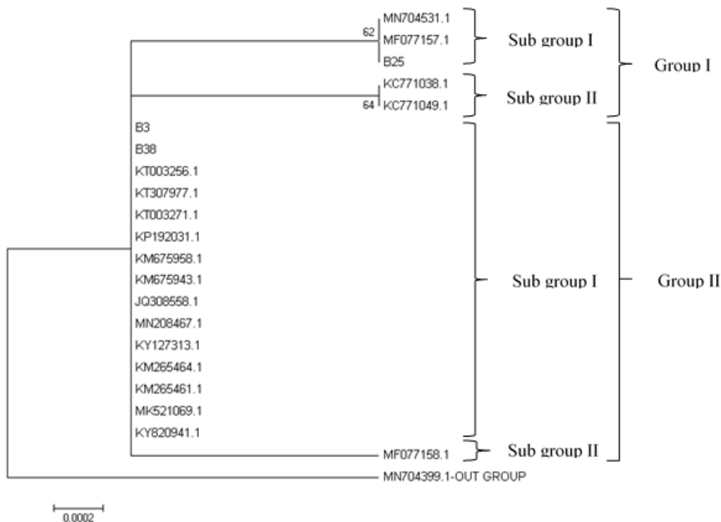
شکل ۵- درخت فیلوژنتیکی حاصل از آنالیز توالی‌های نوکلئوتیدی ناحیه ژنی 16S rDNA در جدایه‌های B3، B25 و B38 باسیلوس با استفاده از الگوریتم Neighbor-joining و مدل p-distance با bootstrap ۱۰۰۰ تکرار انجام شد. از توالی نوکلئوتیدی Bacillus safensis (MN704399.1) به‌عنوان گروه خارجی در فیلوگرام استفاده گردید.
