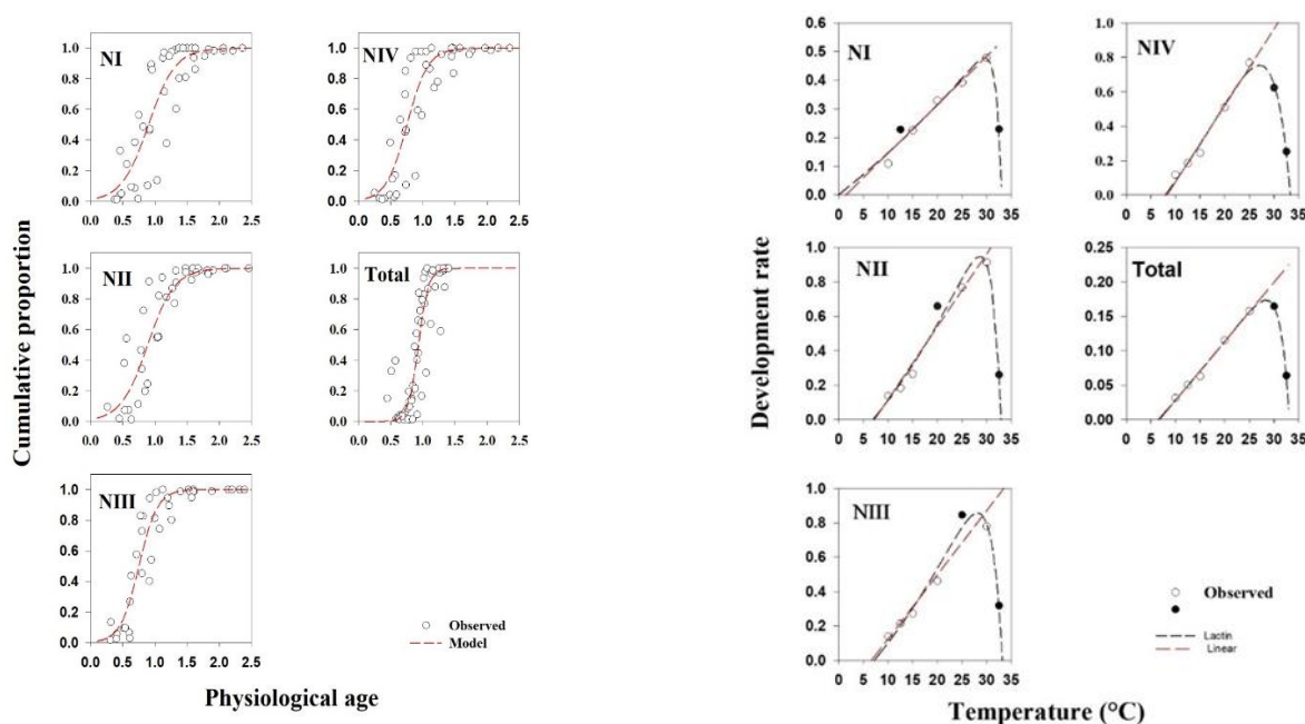
شکل ۱- منحنی نرخ رشد خطی و غیرخطی برای سنین مختلف پورگی و مجموع طول دوره پورگی شته معمولی گندم Scizaphis graminum به‌عنوان تابعی از دما. نقاط داده دایره پر در تحلیل رگرسیون خطی حذف شدند.
